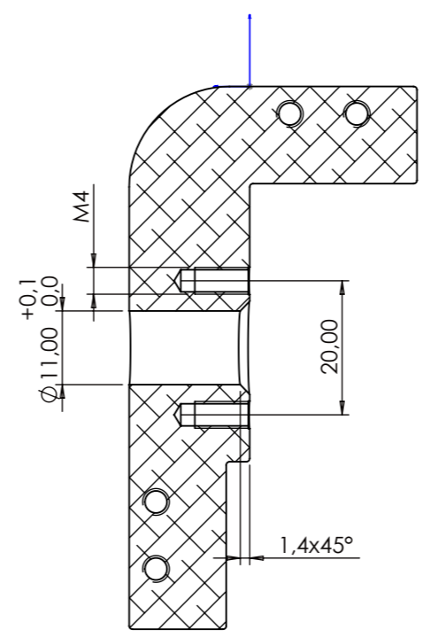
SEZIONE A-A
