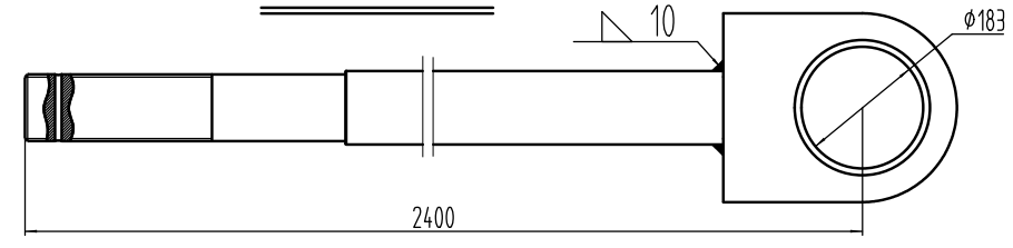
右立柱安装示意图
