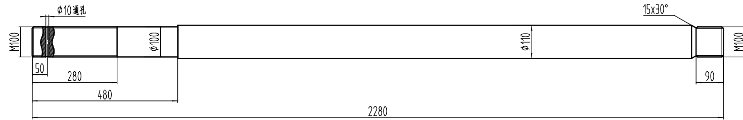
右立柱
