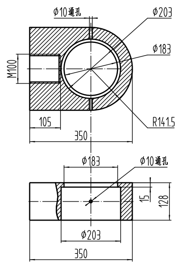
立柱支座
