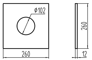
吊梁垫板
