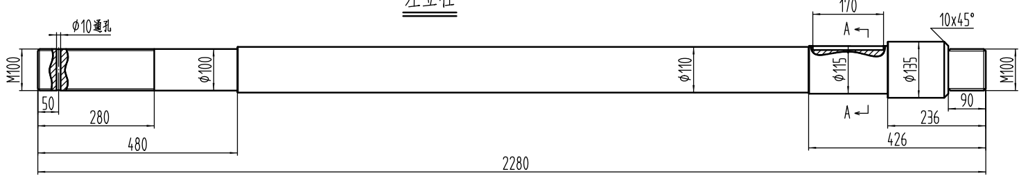
右立柱
