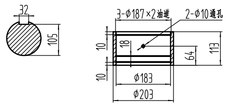
吊梁垫板
