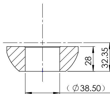
剖面 A-A
