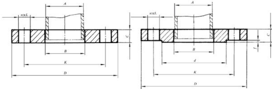
平面(F F )板式平焊钢制管法兰
