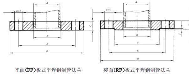
平面(F F )板式平焊钢制管法兰
